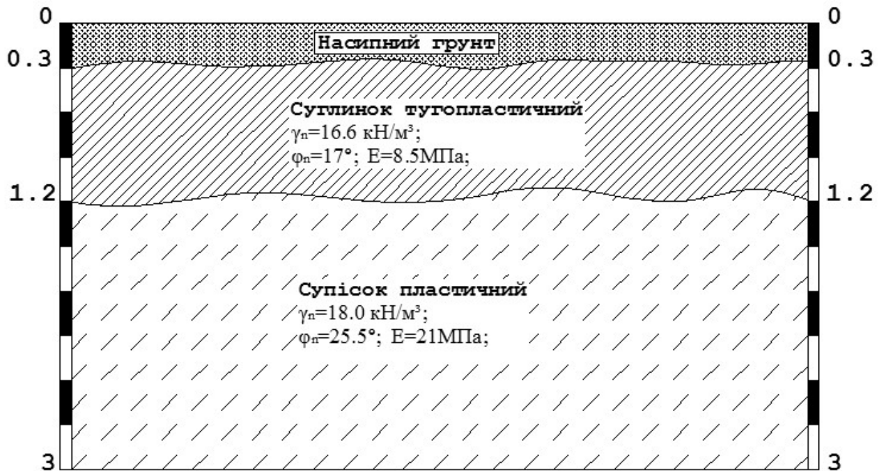
Рис.1 Інженерно-геологічний розріз ділянки випробувань дослідних зразків буронабивних залізобетонних мікропаль
